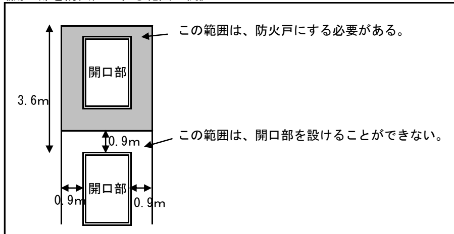
《開口部を防火戸にする範囲の例》
