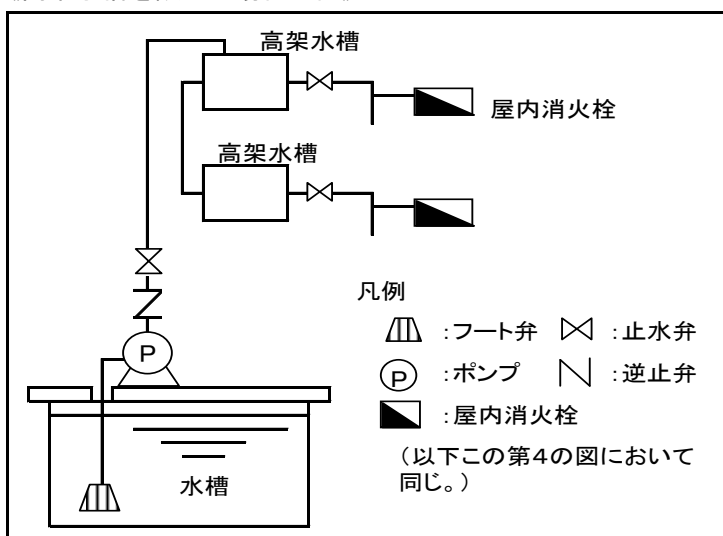
《高架水槽を設けた場合の例》
