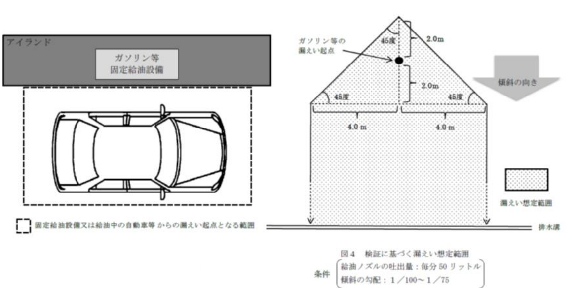
第 3 漏えい起点となる範囲
