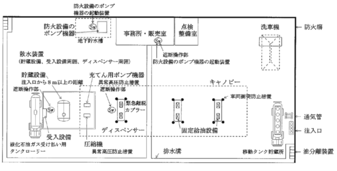
第 2 - 1 液化石油ガス充填設備設置給油取扱所モデル図
