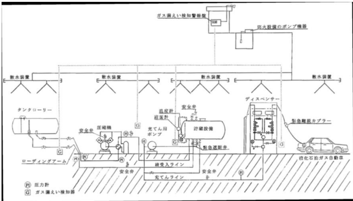
第 2-1 液化石油ガススタンドの概要図 (例)
