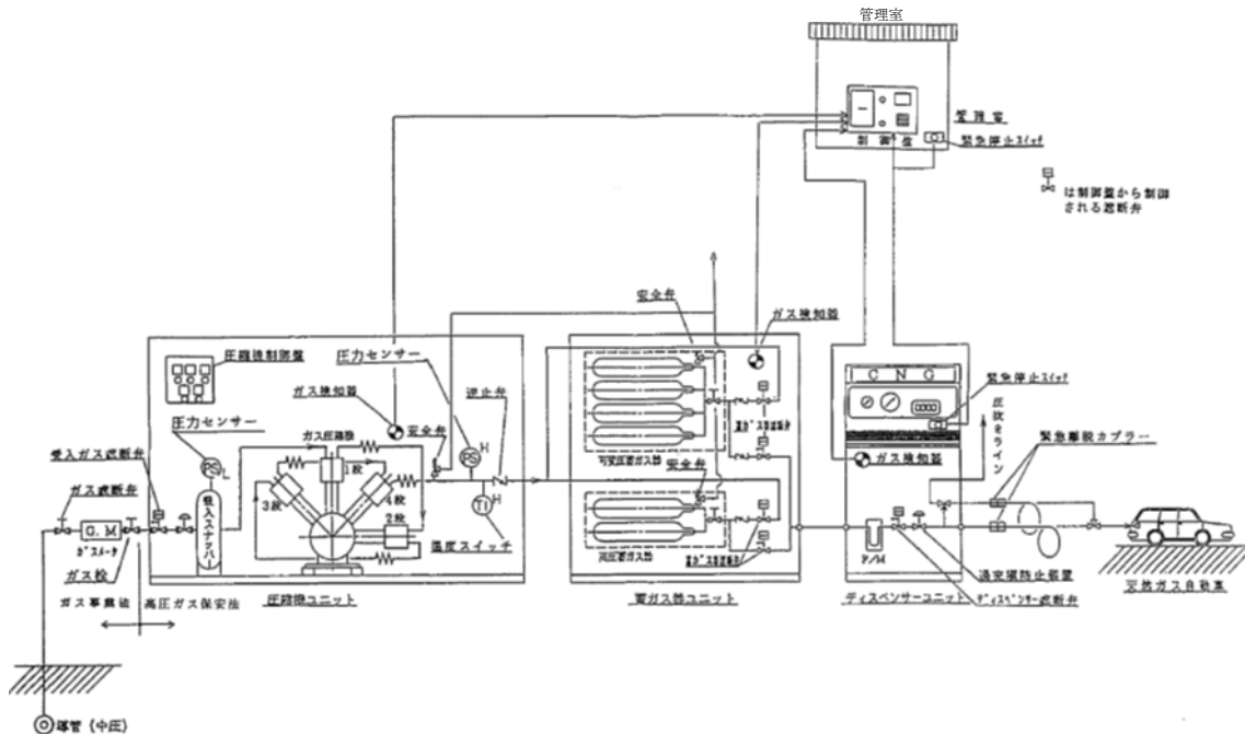
第 1 - 2 圧縮天然ガススタンドの概要図 (例)
