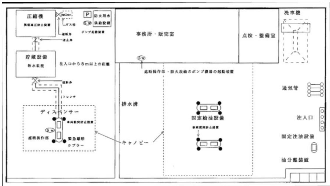
1 - 1 圧縮天然ガス等充填設備設置給油取扱所のモデル図
