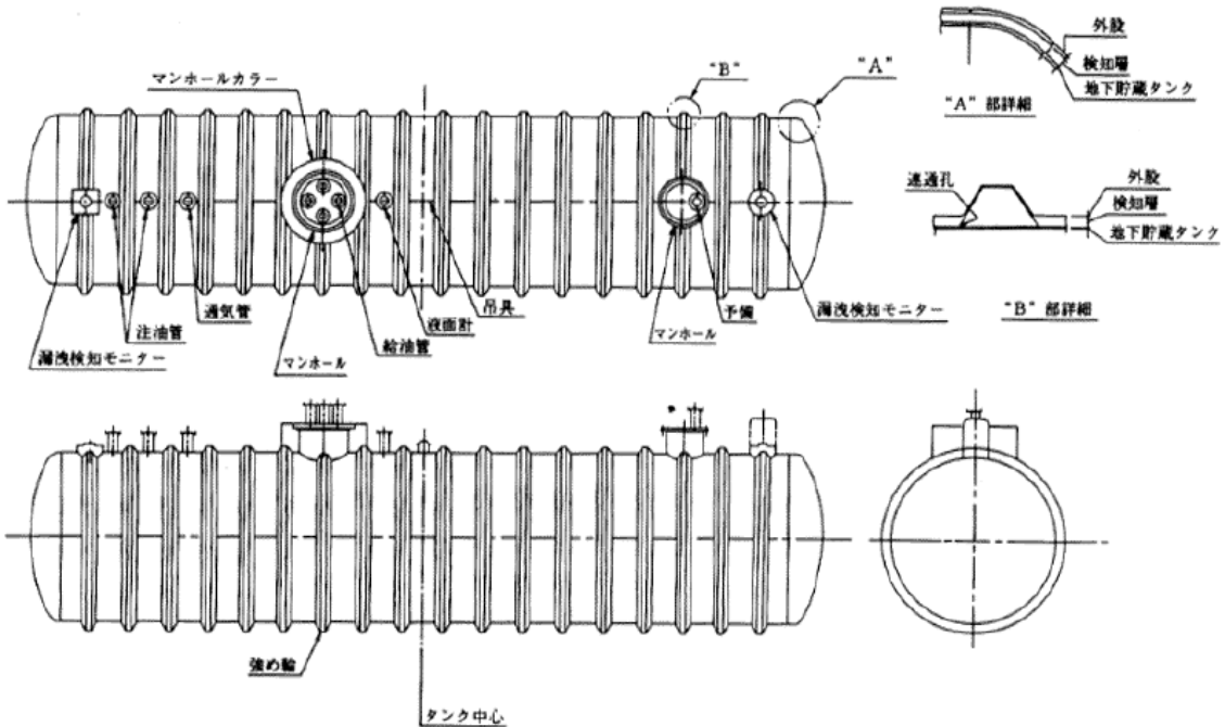
別図一1 強化プラスチック製二重殻タンクの構造例
