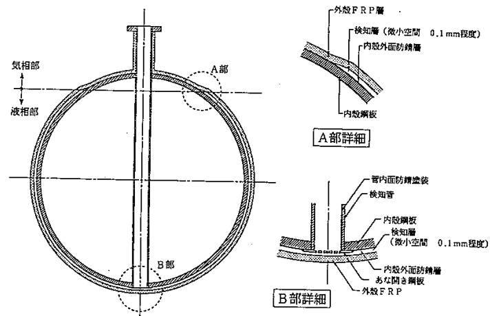
別図一 鋼製強化プラスチック製二重殻タンクの構造例
