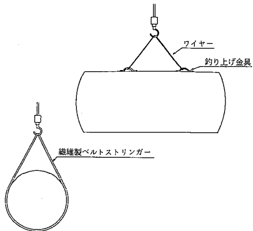
別図二（その1）吊り下げ作業法の例
