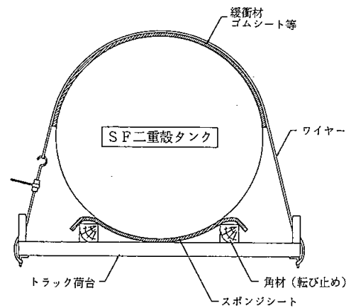
別図二（その2）運搬方法の例
