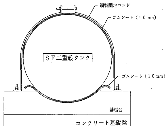
別図三 設置方法の例
