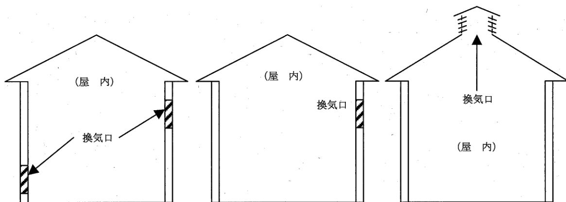
第1-4-1図 自然換気設備の例
