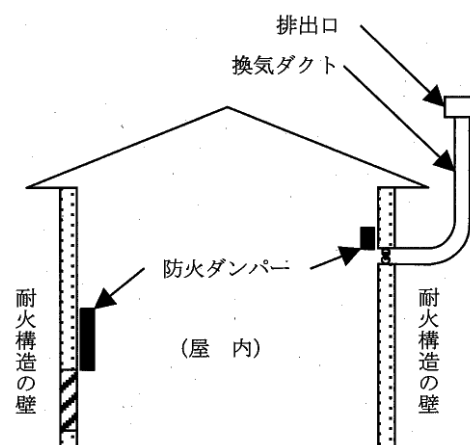
第1-4-6図 防火ダンパーの設置例
