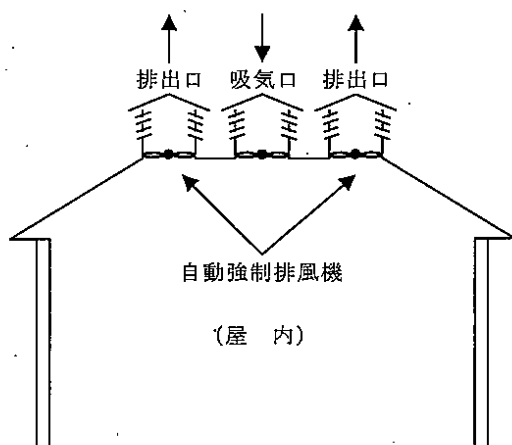
第1-4-5図 自動強制換気設備の例
