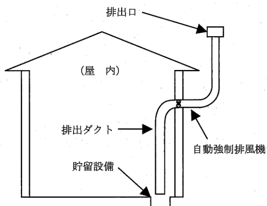
第1-4-8図 自動強制排出設備の例
