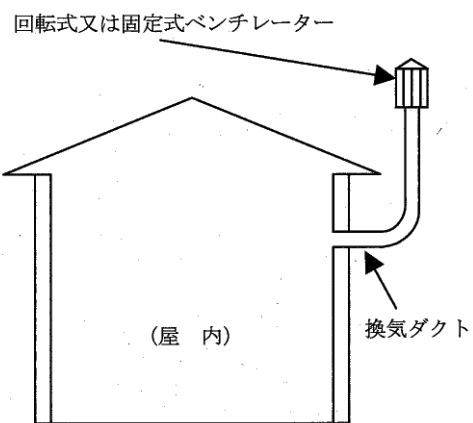
第1-4-3図 強制換気設備の例
