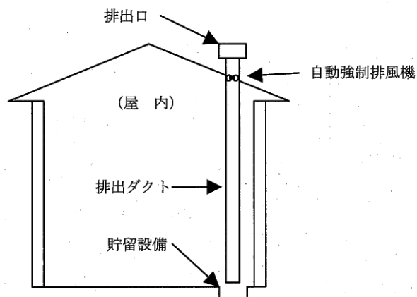
第1-4-9図 自動強制排出設備の例
