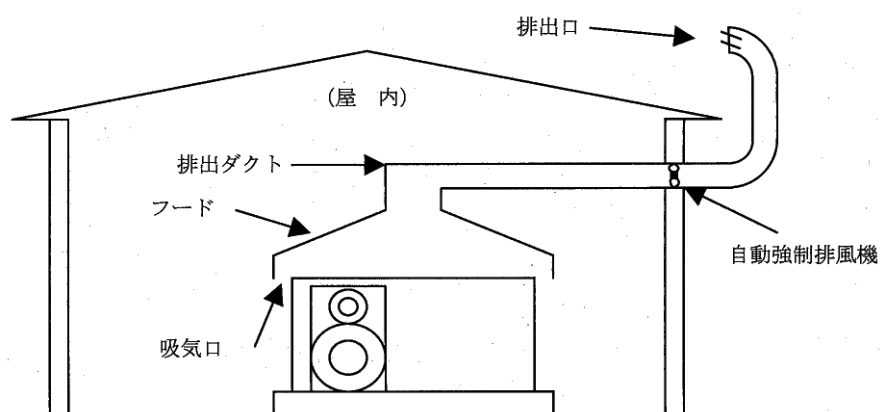
第1-4-7図 自動強制排出設備の例
