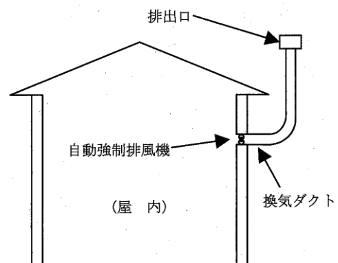
第1-4-4図 自動強制換気設備の例
