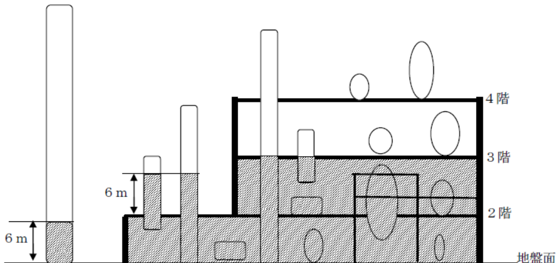
第2-13-1図（2階とみなされる部分の例図）
