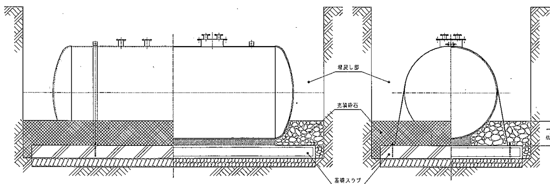
图 3-2. 充填碎石施工图
